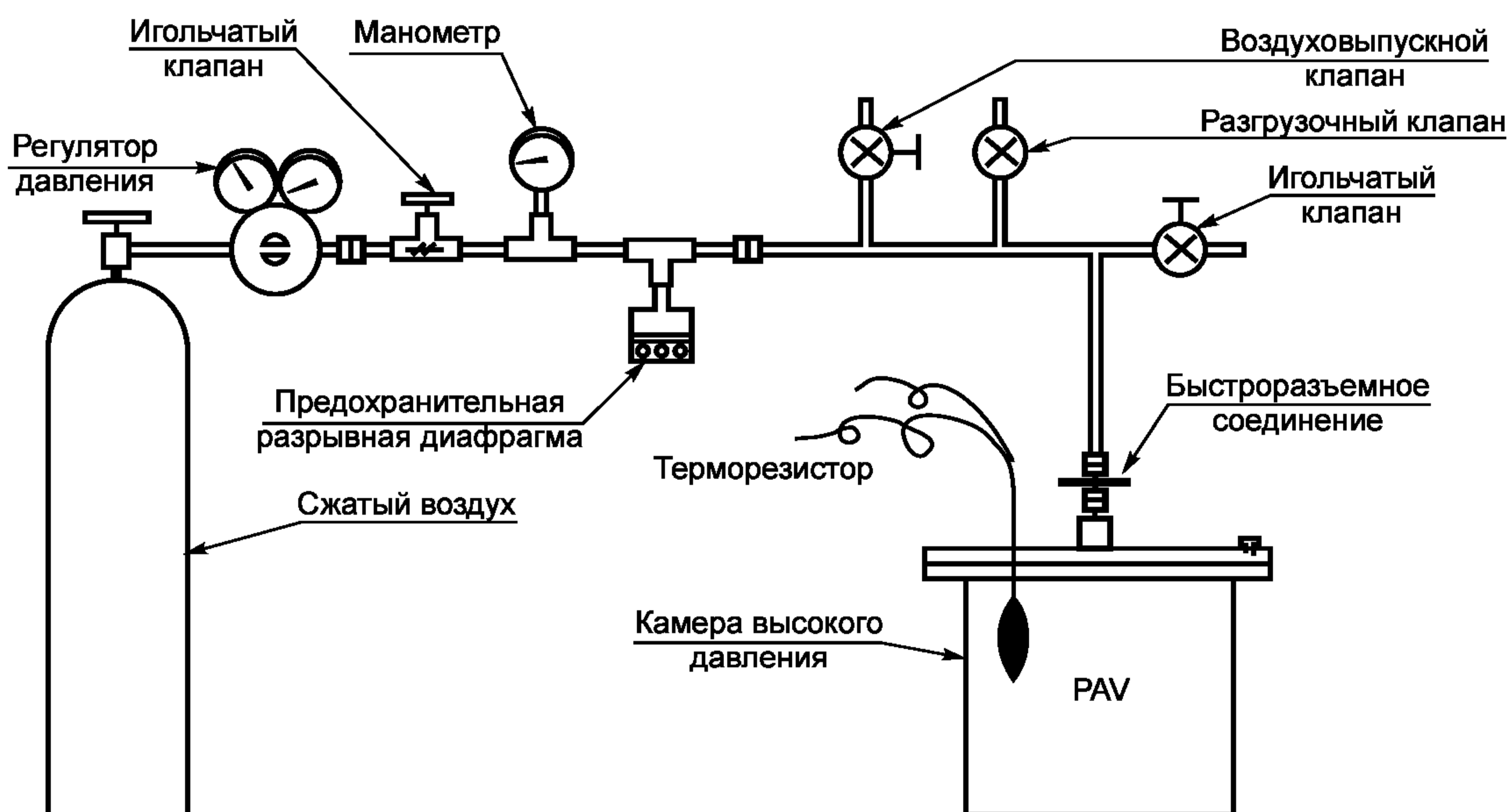
Рисунок 1 — Схема испытательного оборудования
