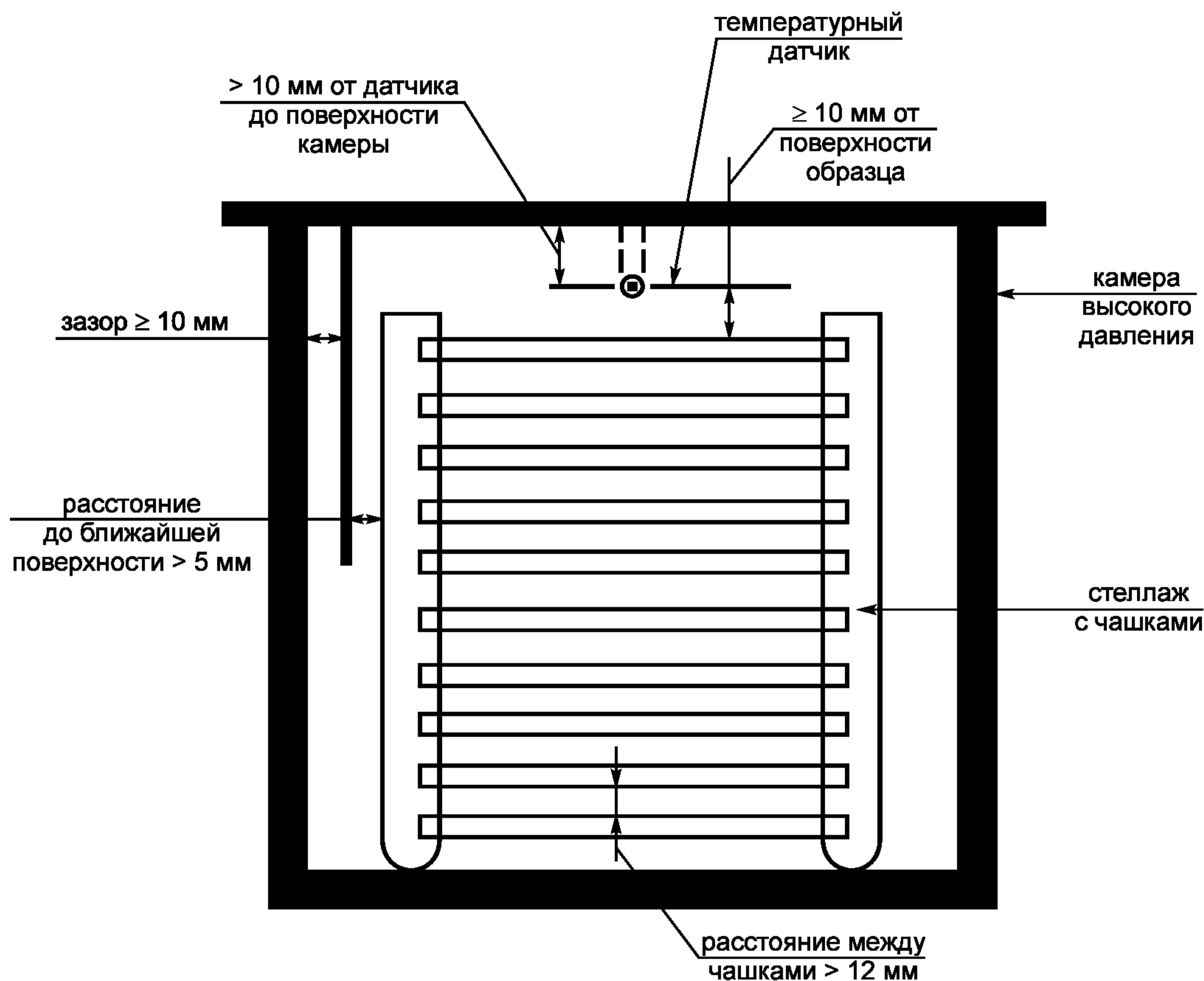
Рисунок 2 — Схема камеры высокого давления
